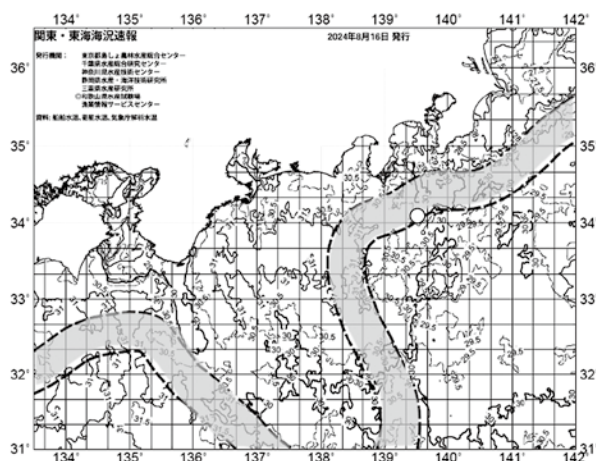
図1 黒潮の流路(島しょセンターHPより) ○が三宅島
