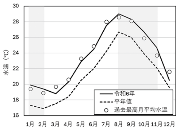
図2 阿古漁港の月平均水温の推移
